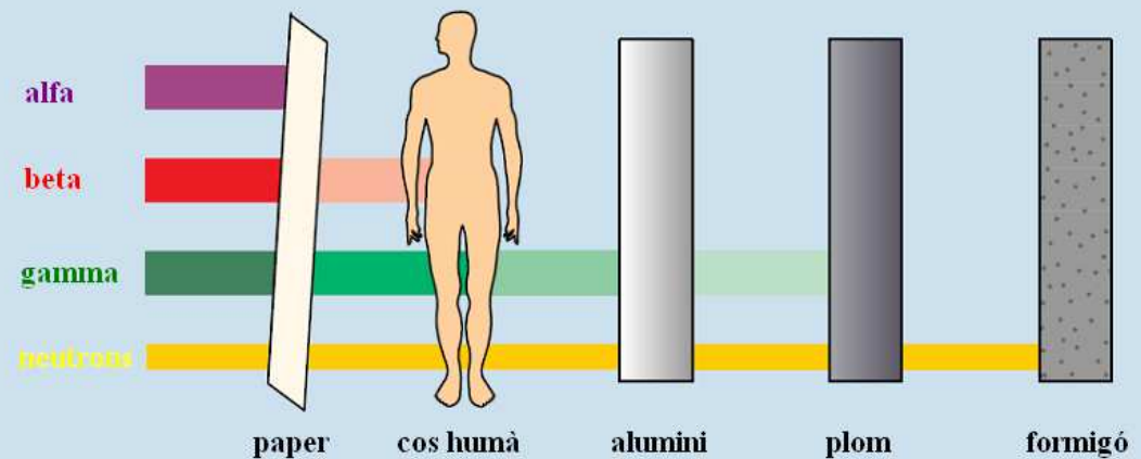
Capacitat de penetració dels diferents tipus de radiació en la matèria
