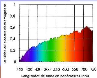
Espectro cromático luz del sol por la tarde
