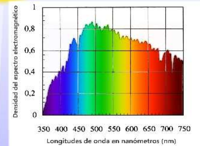
Espectro cromático luz del sol antes del mediodía
