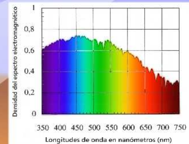
Espectro cromático luz del sol por la mañana
