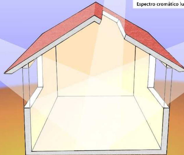
Espectro cromático luz del sol antes del mediodía
